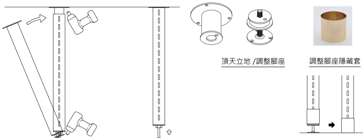
施工範例
